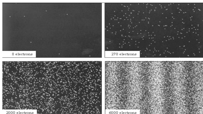
Hình 6. Bức tranh “giao thoa” của electron trong thí nghiệm khe Young
