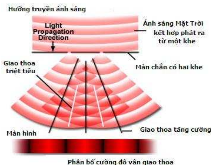
Hình 4. Mô hình hiện tượng “giao thoa” của ánh sáng
