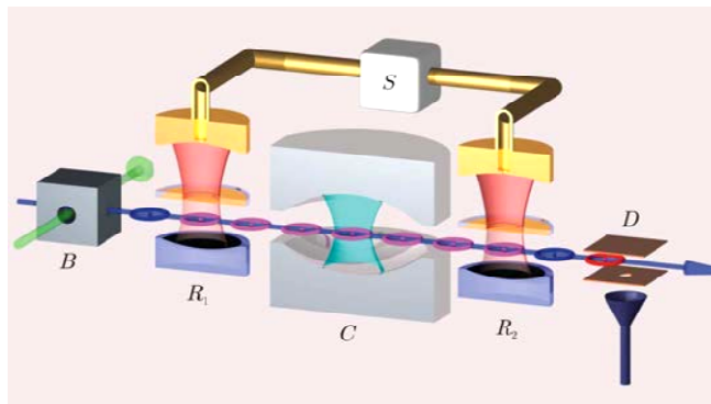
Sơ đồ bố trí thí nghiệm điều khiển và đo lường hạt photon đơn lẻ bằng bẫy nguyên tử Rít-bóc
